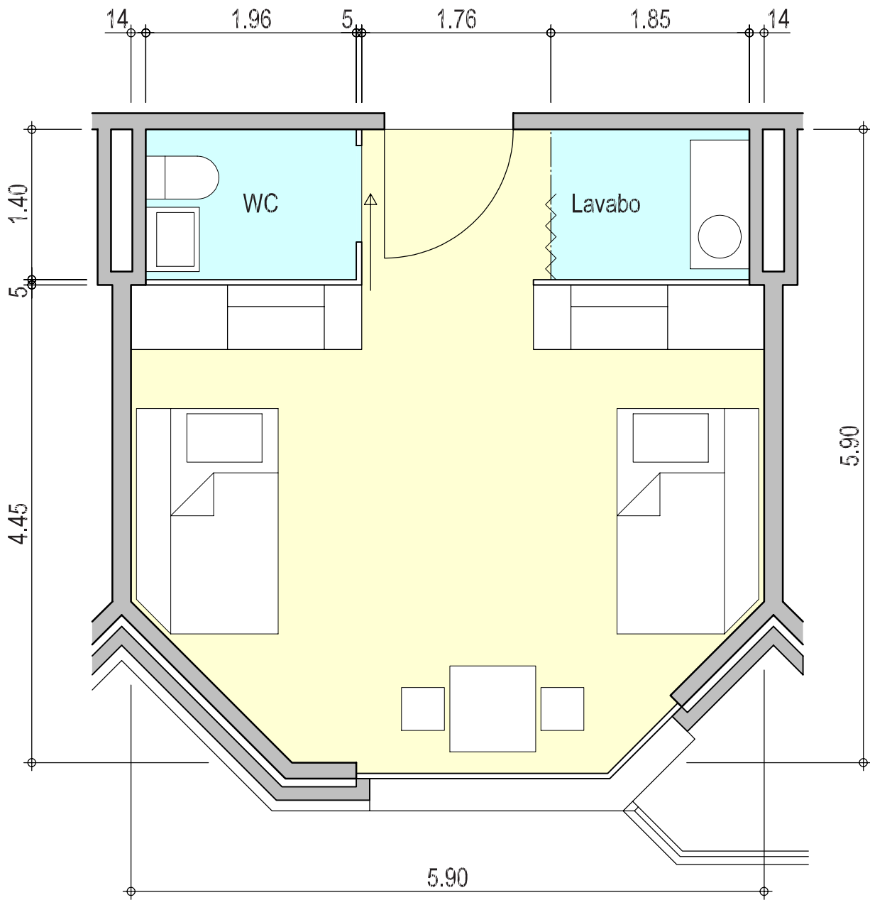
2-Bett-Pflegezimmer 32.7 m 2
