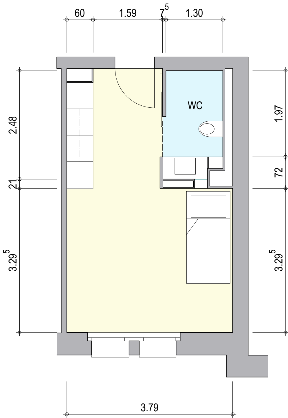
Pflegezimmer 21.5 m 2
